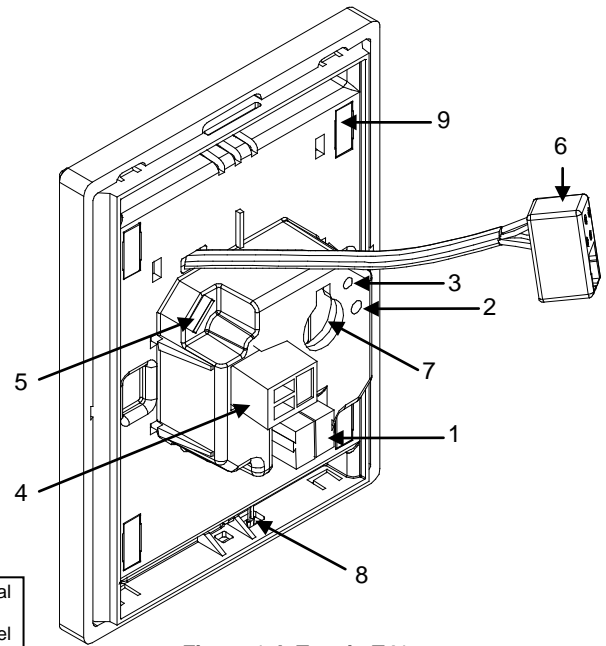
Figura 1. InZennio Z41
